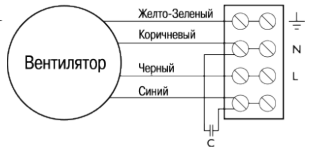
Схема № 2 ~230 В, 1 фаза
